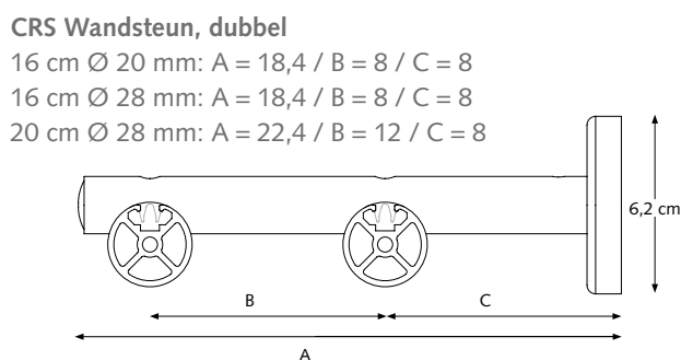
CRS Wandsteen, dubbel 16 cm Ø 20/28 mm
